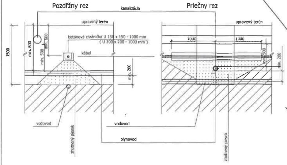
Križovanie plynovodu s káblami NN, VN, TLF a vodovodu
